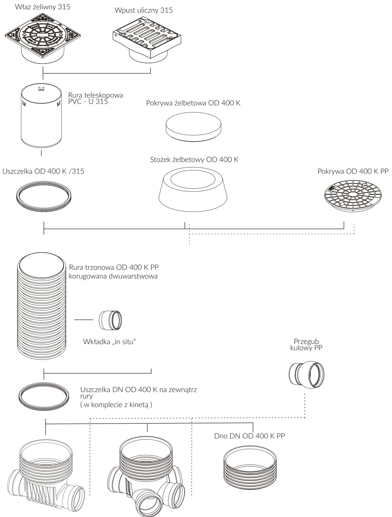
Kineta przelotowa OD 400 K PP Kineta zbiorcza OD 400 K PP
